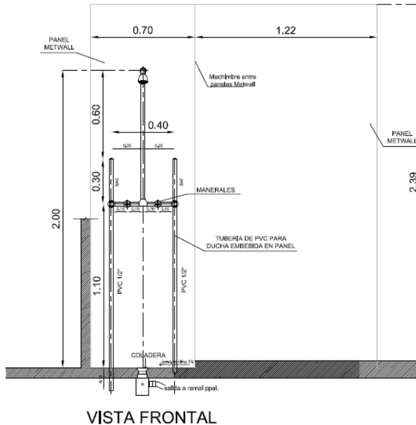
Instalación para Ducha Fig. 10
